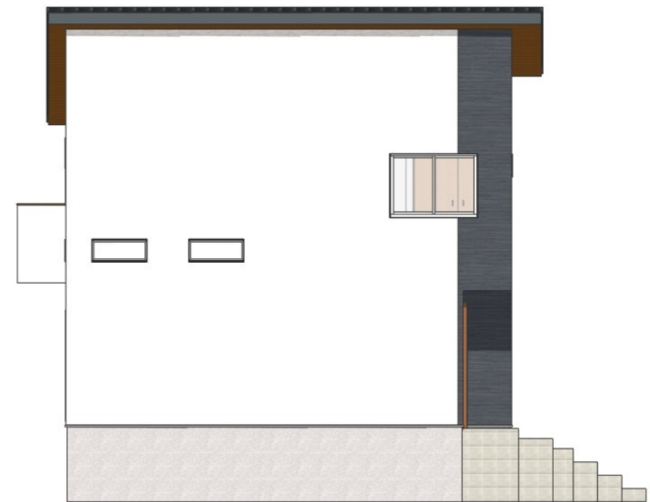
東立面図
