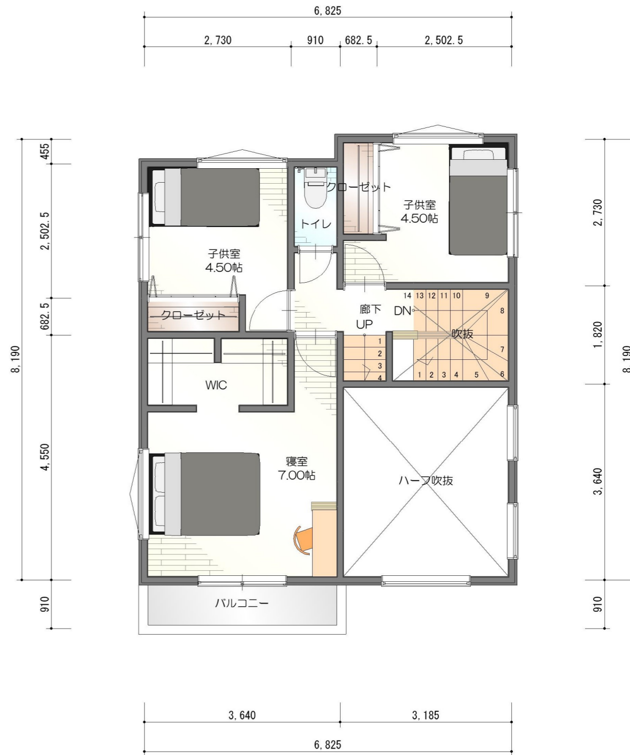
2階平面図
